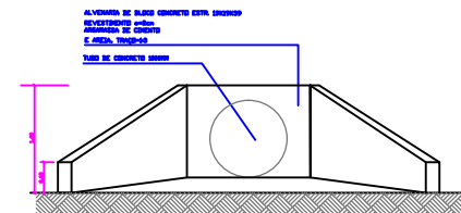
ALA VISTA Escala 1:5
