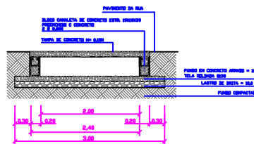
GALERIA CORTE TRANSVERSAL Escala 1:5
