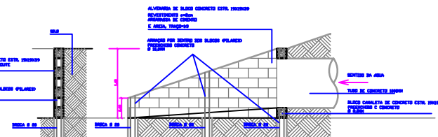
ALA CORTE TRANSVERSAL E LONGITUDINAL Escala 1:5
